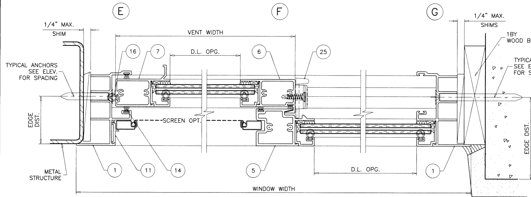
XO LAYOUT
